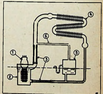
Fig. 12. Het koelsysteem van de „Vapotron”. 1 — Vapotron; 2 — kookketel; 3 — isolatiebuizen van pyrex; 4 — condenser; 5 — reservoir; 6 — drukregelaar.
