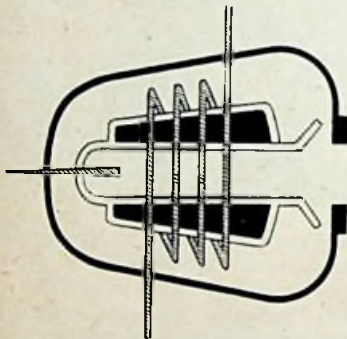
Fig. 8. Schematiek van de ionofoon
