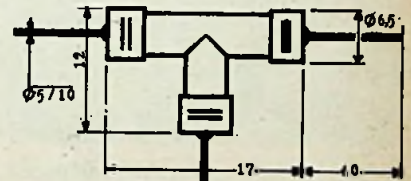
Fig. 10. Germanium kristaltriode van Westinghouse.
