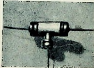
Fig. 10. Germanium kristaltriode van Westinghouse.
