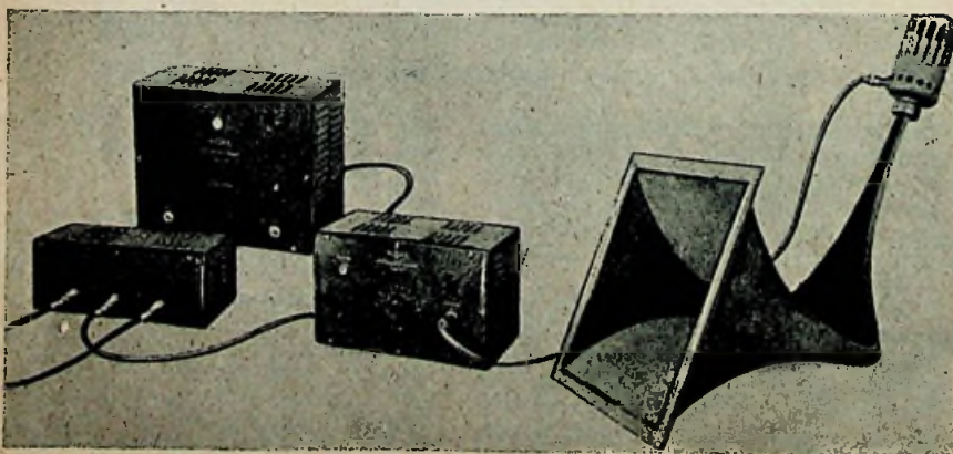
Fig. 9. De commerciële ionofoon bij „Audax”. De complete installatie (20.000—200 Hz).
