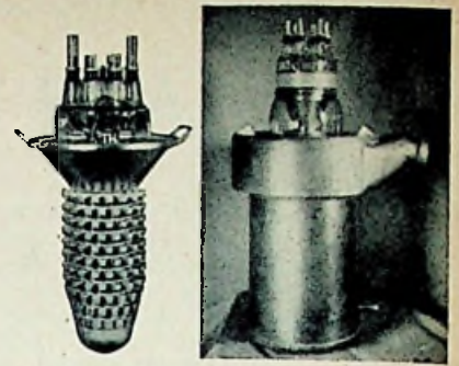
Fig. 11. De „Vapotron” van Thomson-Houston, een zendbuis met 3-voudig rendement. Rechts: in de „pan”.
